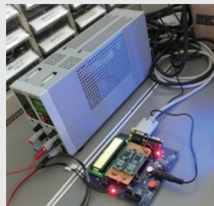
図5 統一電源プラグ・システムの試作機
