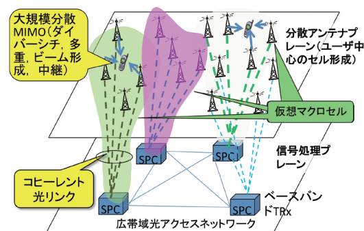
図2 分散アンテナネットワーク
