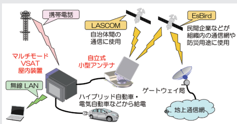
図1 今回開発したマルチモード VSAT を用いたシステムの概要
