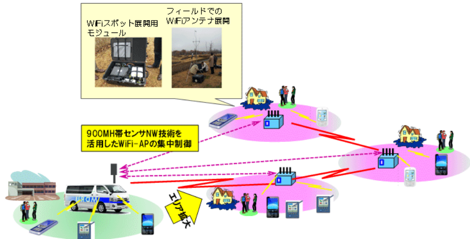
図:ICTカーによる被災地でのWi-Fiエリア化
