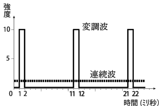
図2 変調：連続波と変調波
