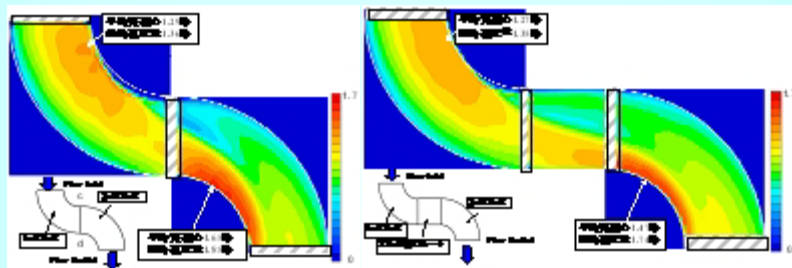
PIVシステムによる テュアルエルボ内流動可視化結果
