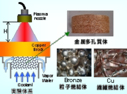
金属多孔質体を用いた超高温熱流束除去技術の開発
