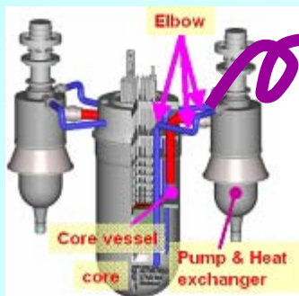
次世代高速炉
