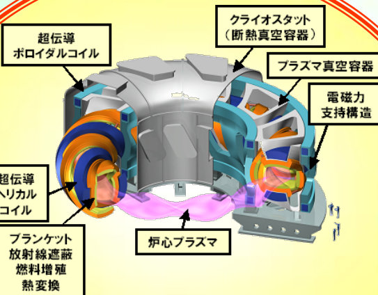
ヘリカル型発電実証炉 FFHR
