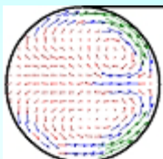
断面内二次流れ
