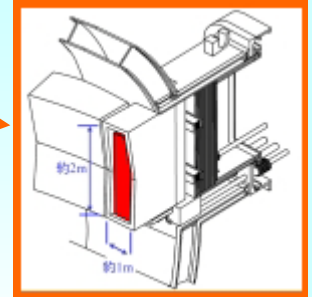
TBM用先進液体ブランケットの設計
