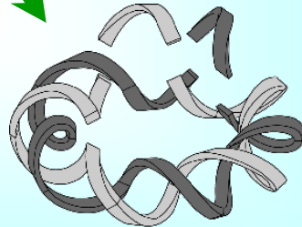
分割型超伝導マグネット設計
