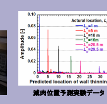
減肉位置予測実験データ
