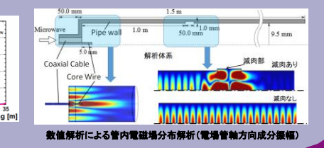
数値解析による管内電磁場分布解析 (電場管軸方向成分振幅)
