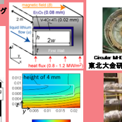
流路内MHD熱流動特性の評価
