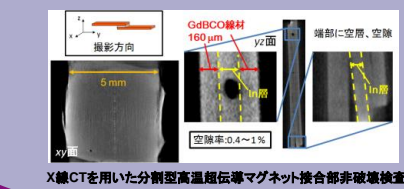
X線CTを用いた分割型高温超伝導マグネット接合部非破壊検査
