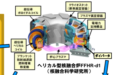
ヘリカル型核融合炉FFHR-d1 (核融合科学研究所)
